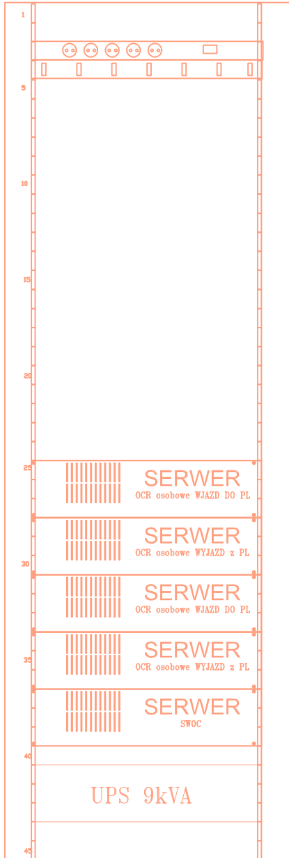
WIDOK PRZÓD
