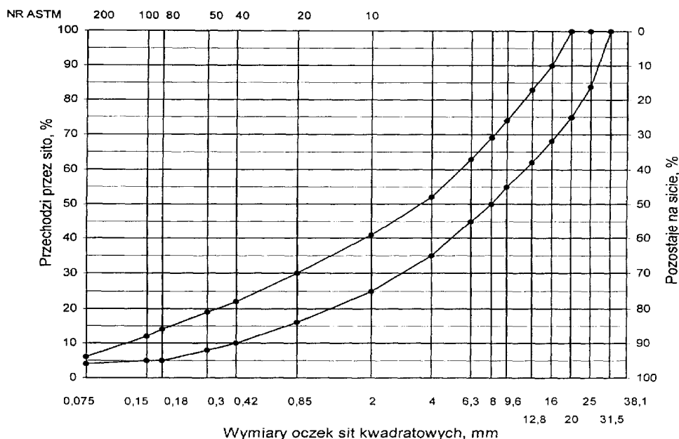
Rys. 1. Krzywe graniczne uziarnienia mieszanki mineralnej BA od 0 do 25 mm do warstwy wiążącej nawierzchni drogi o obciążeniu ruchem KR4
