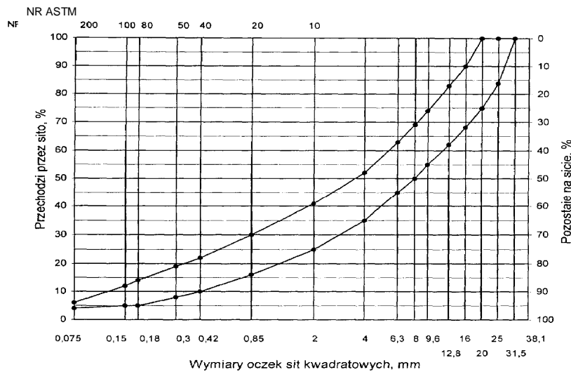
Rys. 12. Krzywe graniczne uziarnienia mieszanki mineralnej BA od 0 do 20 mm do warstwy wiążącej nawierzchni drogi o obciążeniu ruchem od KR3 do KR6
