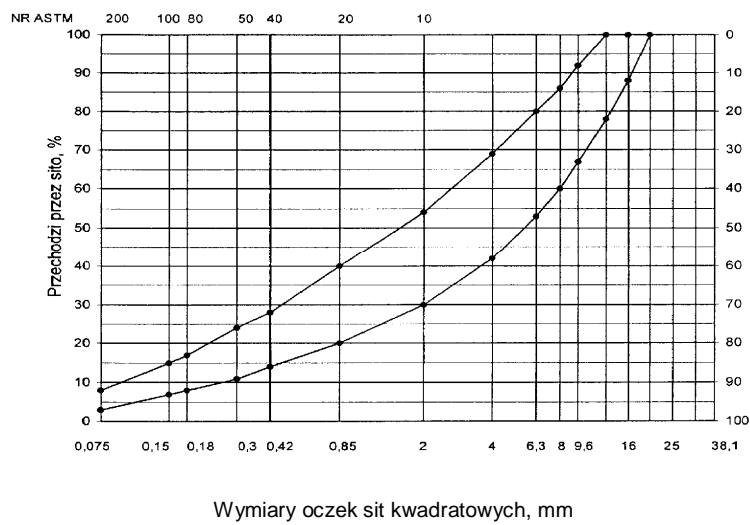
Rys. 9. Krzywe graniczne uziarnienia mieszanki mineralnej BA od 0 do 16 mm do warstwy wiążącej nawierzchni drogi o obciążeniu ruchem KR1 lub KR2
