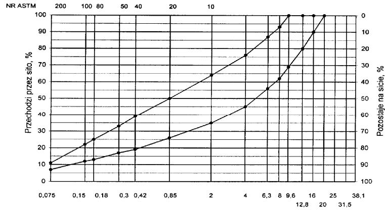
Wymiary oczek sit kwadratowych, mm
