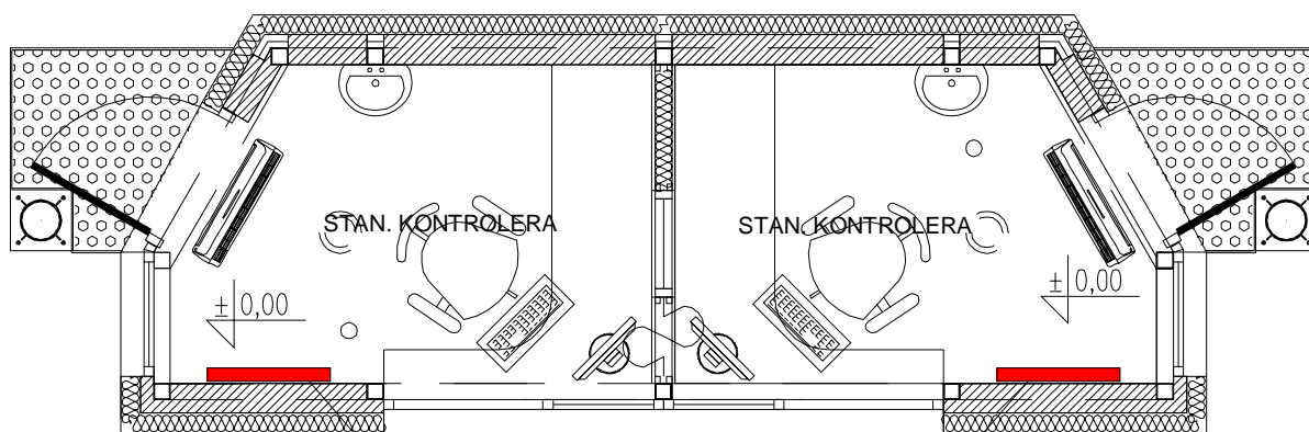
GRZEJNIK ELEKTRYCZNY ATLANTIC TYP F117 O MOCY 2,0kW
