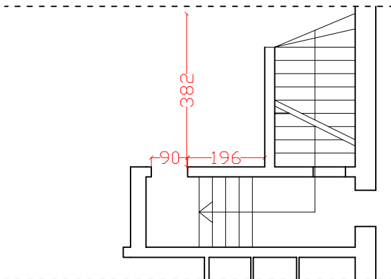
Rzut parteru
