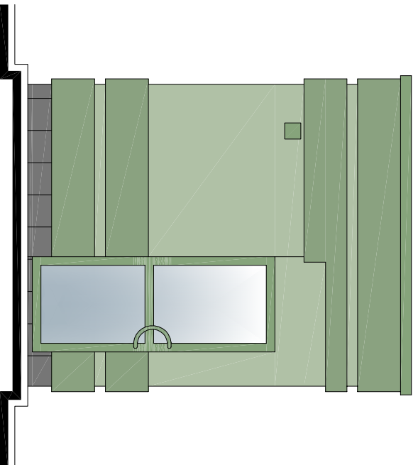
ELEWACJA BOCZNA 1:50
