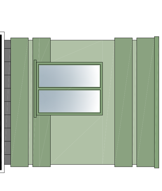
ELEWACJA BOCZNA 1:50
