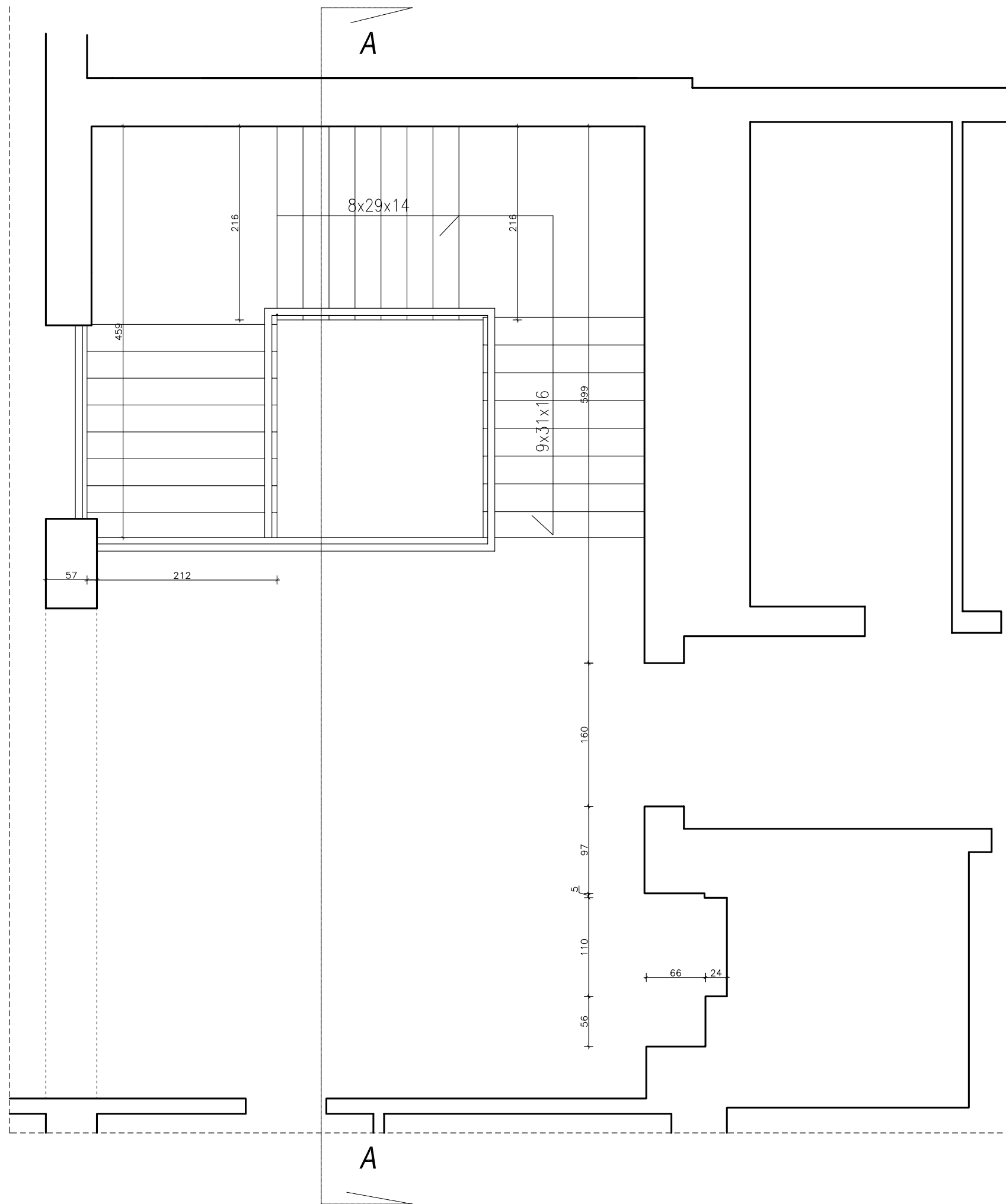
Rzut 3-go piętra
